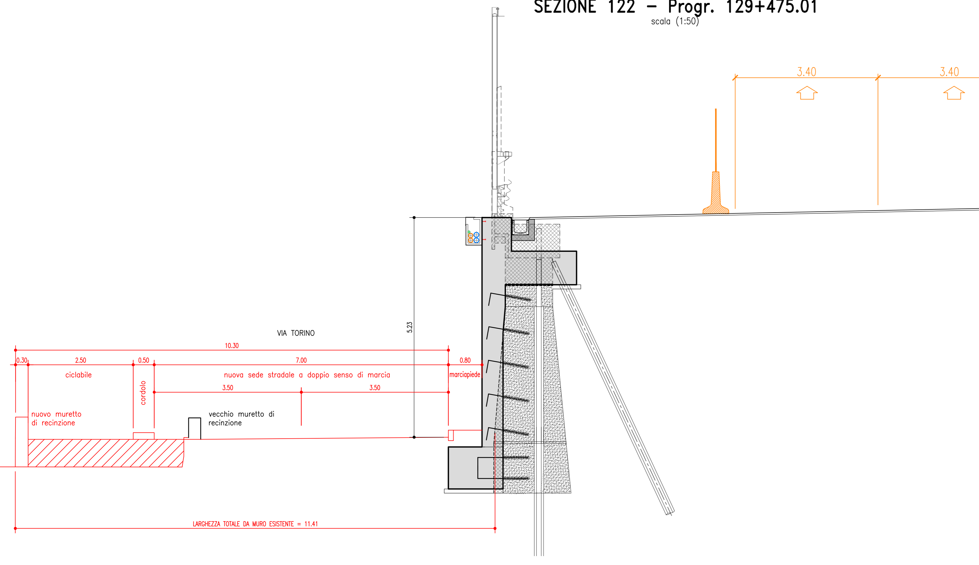
SEZIONE 122 - Progr. 129+475.01
