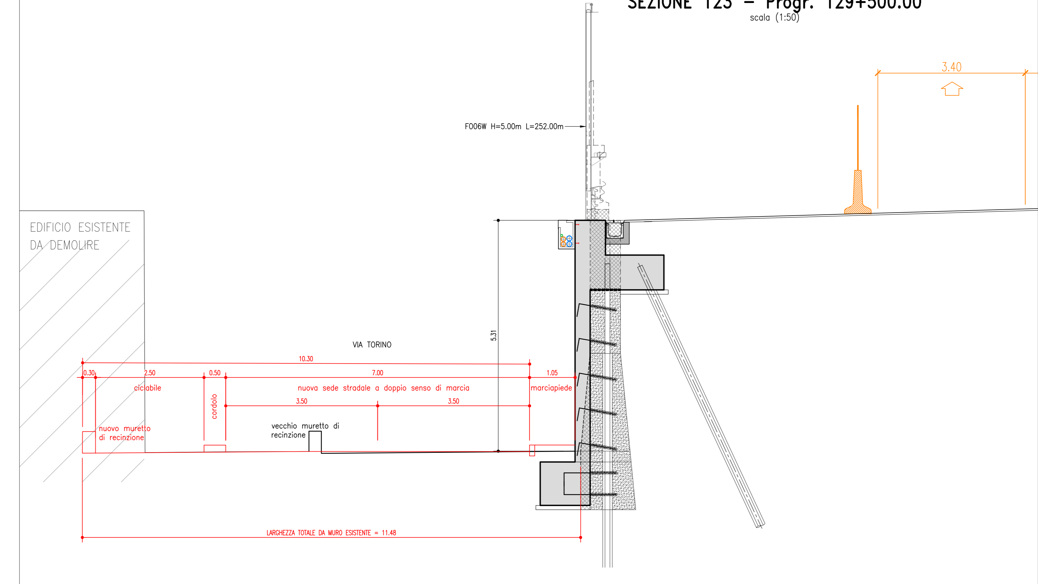
SEZIONE 123 - Progr. 129+500.00
